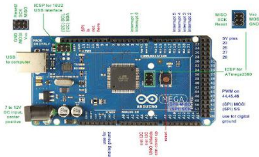
Gambar 2.2 Mikrokontroler Arduino Mega2560
