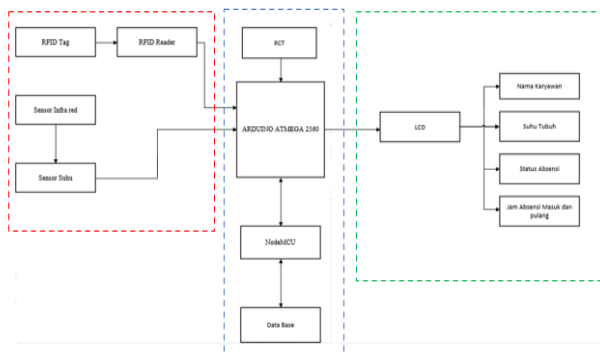
Gambar 3.2 Diagram Blok
