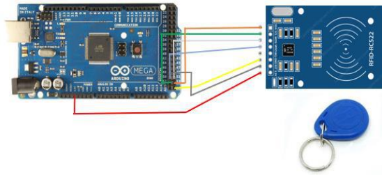
Gambar 3.4 Rangkaian RFID
