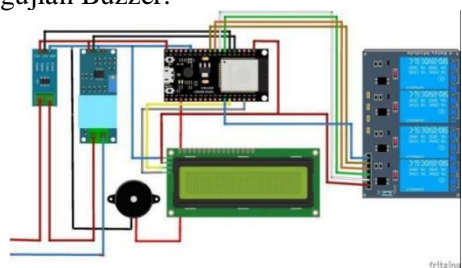
Gambar 12 - Skematik Pengujian Buzzer
