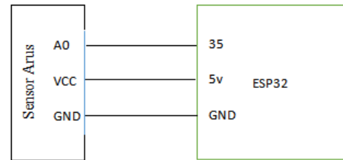
Gambar 7 - Skematik Sensor Arus ACS712
