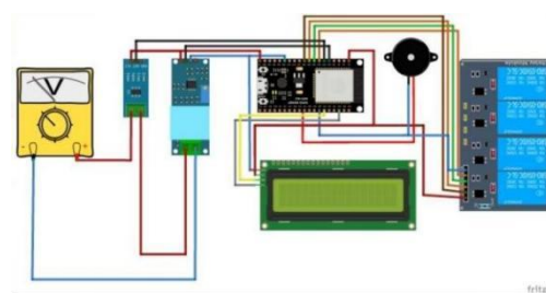
Gambar 11 - Skematik Pengujian Sensor Tegangan
