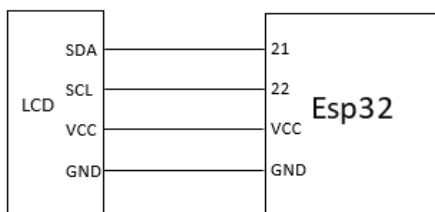
Gambar 5 - Skematik LCD I2C
