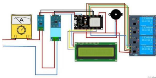
Gambar 10 - Skematik Pengujian Sensor Arus
