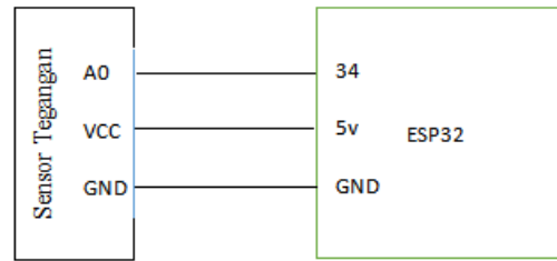
Gambar 6 - Skematik Sensor Tegangan
