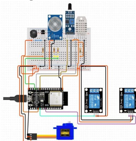
Gambar 3.4 Skema rangkaian sistem
