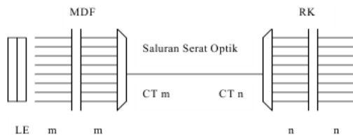
Gambar 2. Konfigurasi Jaringan Digital Loop Carrier
